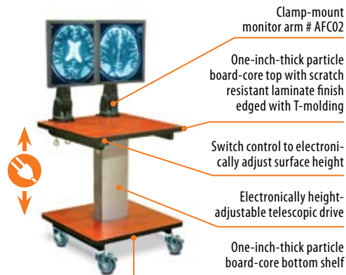
A. Telescopic Cart™ 24"W x 24"D
