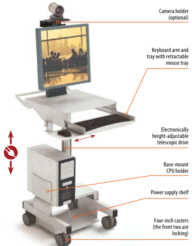
Deluxe PC Cart™ 500
