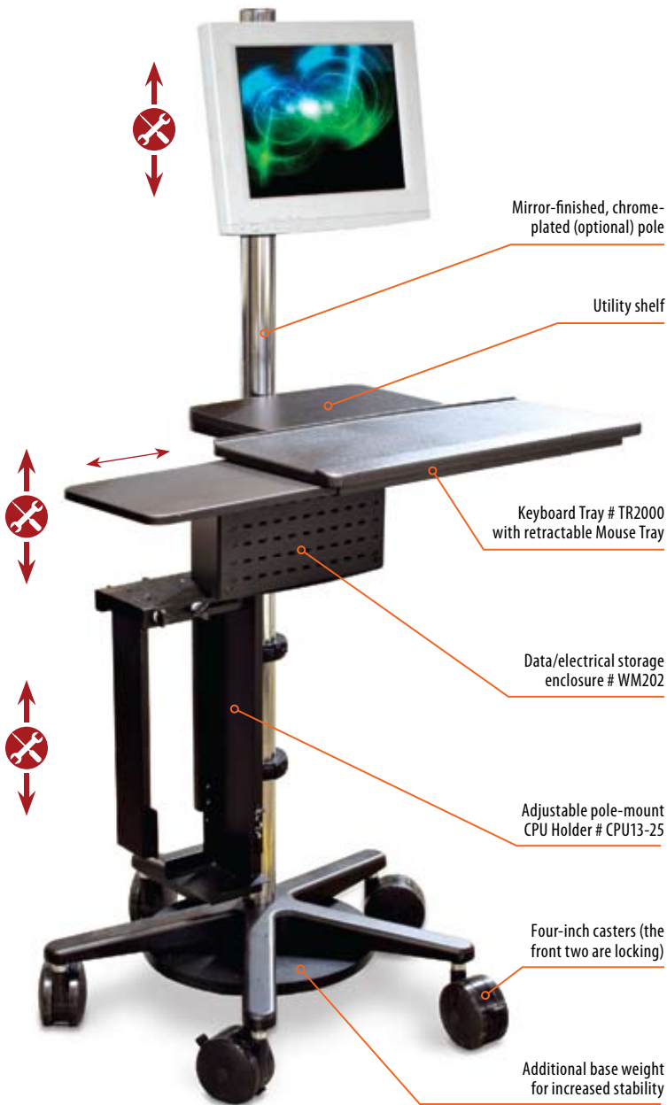
Pole Cart™ MPC200
