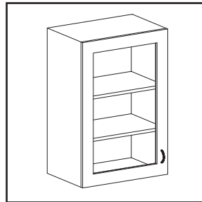
WC 24"W x 16"D x 36"H
